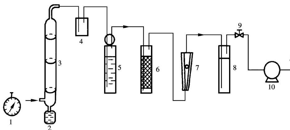
1—秒表；2—皂液；3—皂膜流量计；4—皂液捕集器；5—吸收管（瓶）；
