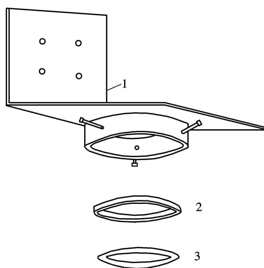
碱片采样架
